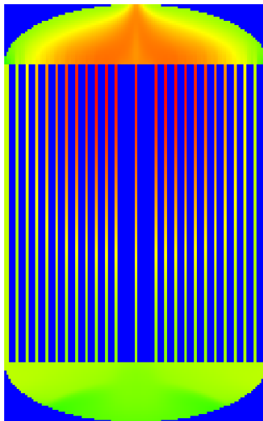
(c) D=10^{-7}\text{m}^2\text{s}^{-1} , groupe 0
