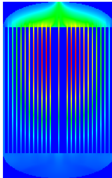
(d) D=10^{-7}\text{m}^2\text{s}^{-1} , ensemble des neutrons retardés
