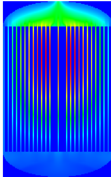
(b) D=10^{-9}\text{m}^2\text{s}^{-1} , ensemble des neutrons retardés
