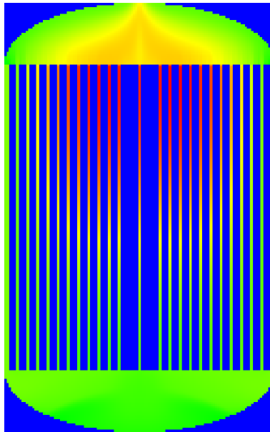
(a) D=10^{-9}\text{m}^2\text{s}^{-1} , groupe 0
